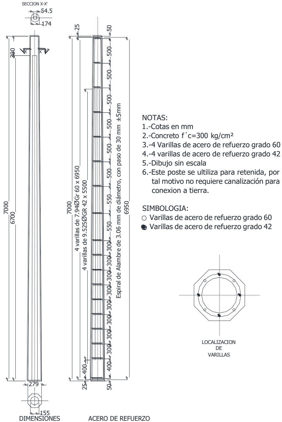
FIGURA 2– Poste PCRGR60-7-500
